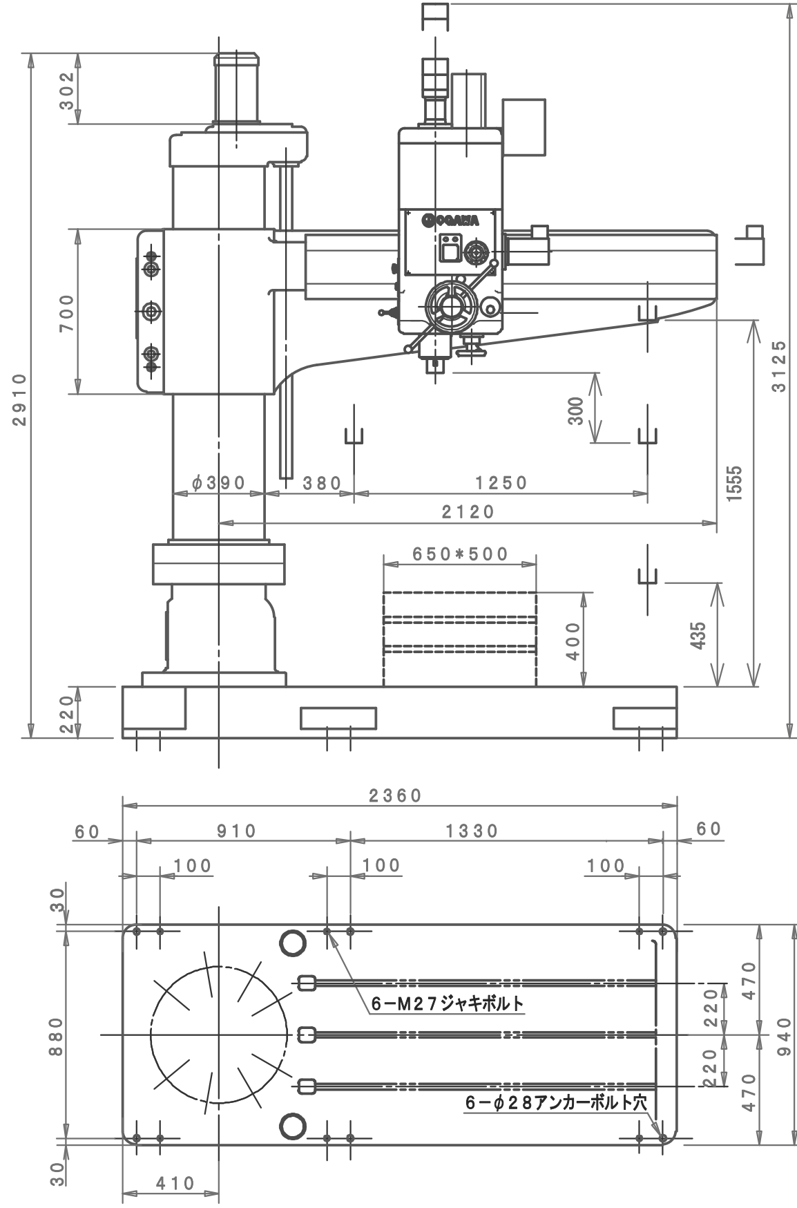
第01.0図 全体図
