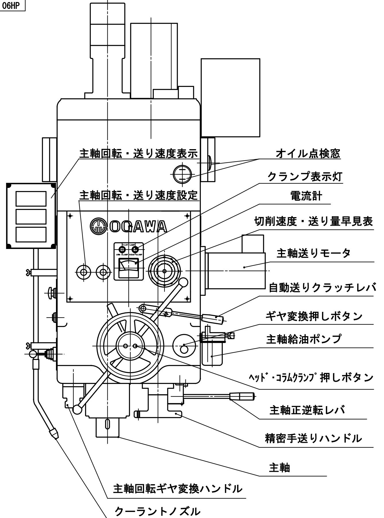
第 2 1 . 2 図 操作部
